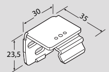
Beugel voor achterzijde montage
