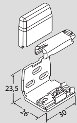
Zijgeleidingsbeugel voor achterzijde montage (optioneel) Type A011
