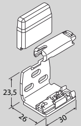
Zijgeleidingsbeugel voor achterzijde montage (optioneel) Type A029
