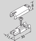
Zijgeleidingsbeugel voor onderzijde montage (optioneel) Type A029
